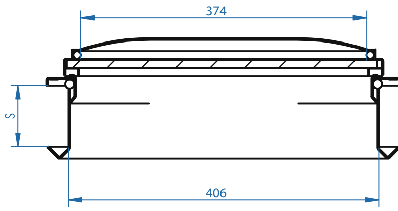
SEZIONE A-A
