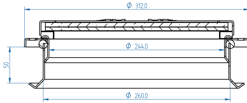
SEZIONE A-A
