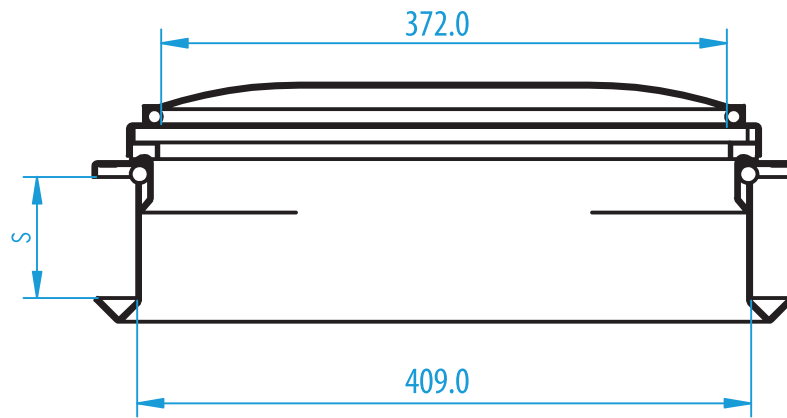
SEZIONE A-A
